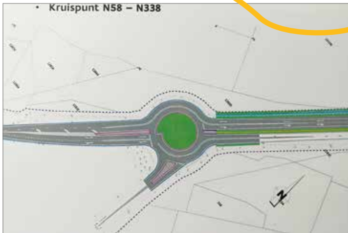
▲ De rotonde met de N338 wordt een turborotonde met voorsorteervakken.
